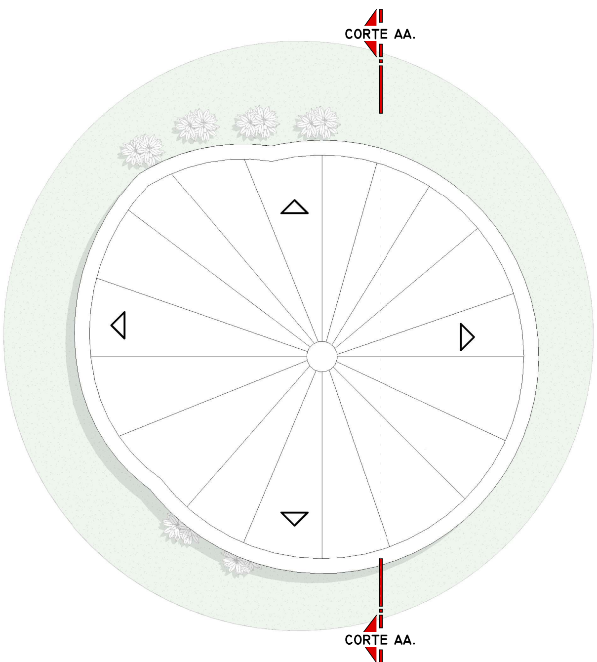
PLANTA DE COBERTURA - BANGALÔ ESC: 1 : 100
