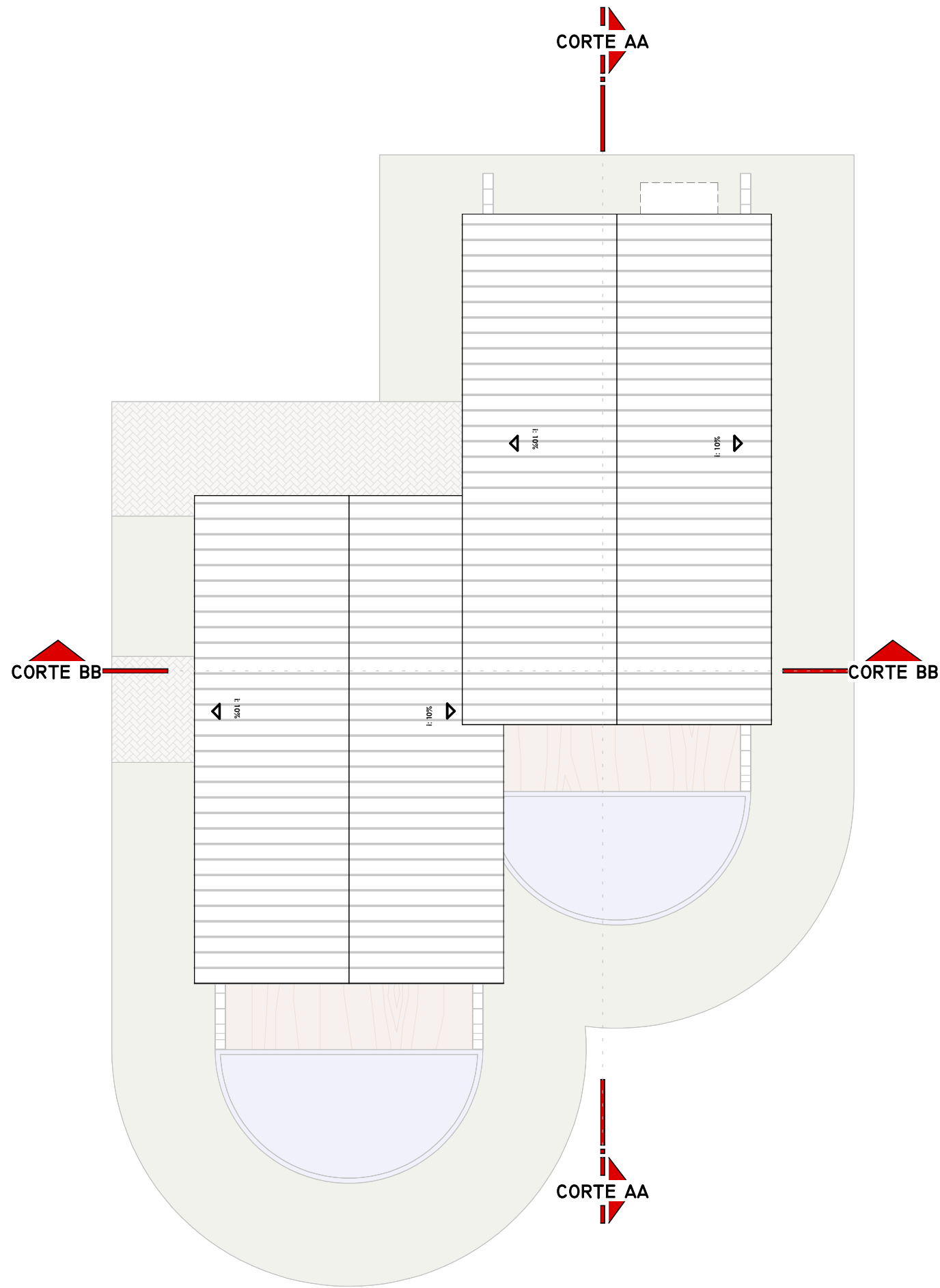
PLANTA DE COBERTURA - APARTAMENTOS ESC: 1 : 100
