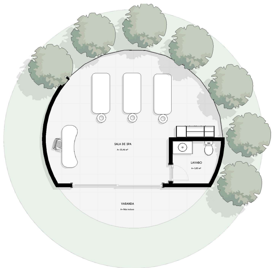
PLANTA BAIXA - SPA ESC: 1 : 100
