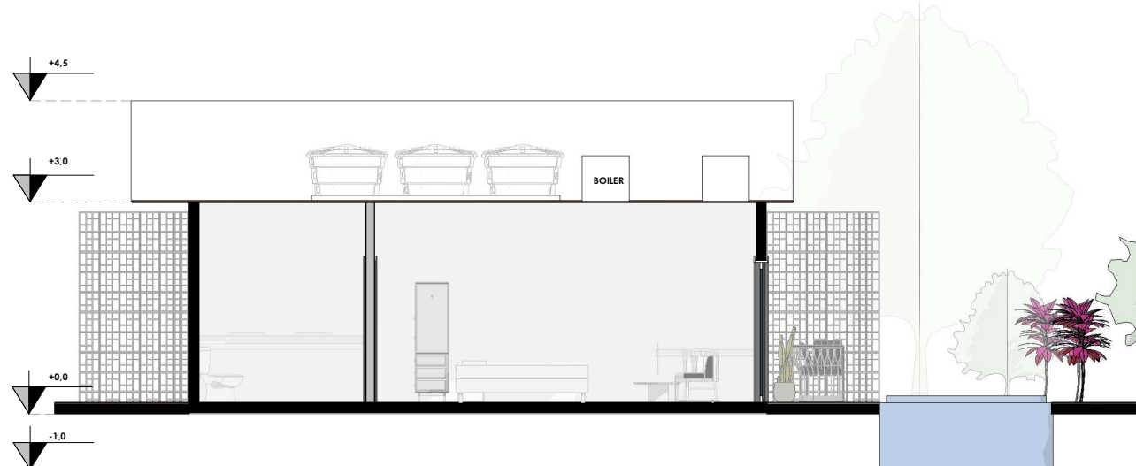
CORTE AA - APARTAMENTO ESC: 1 : 100
